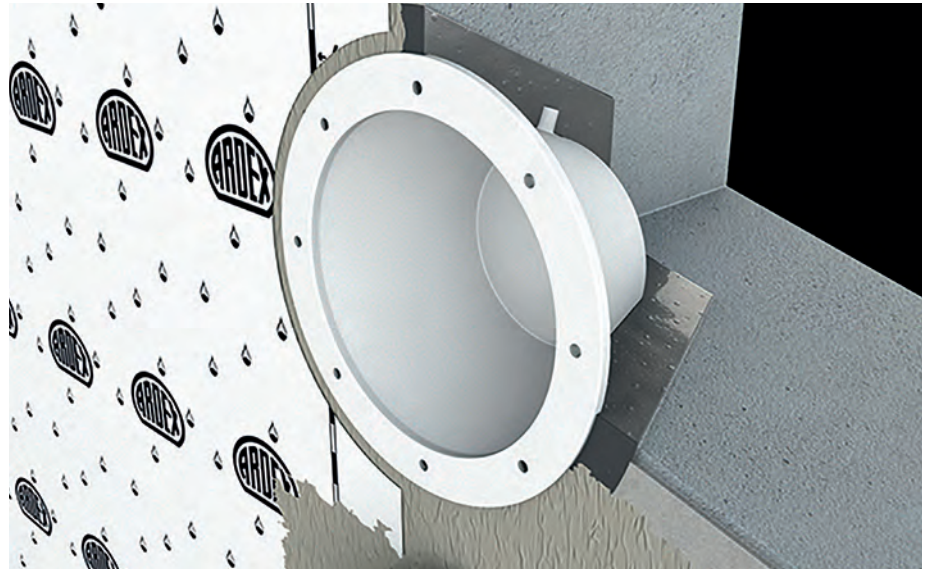
Havuz aydınlatma uygulama kesiti
