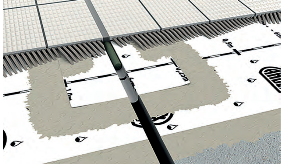
Dilatasyon uygulama kesiti
