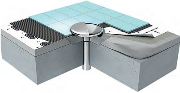
Su gideri uygulama kesiti 2
