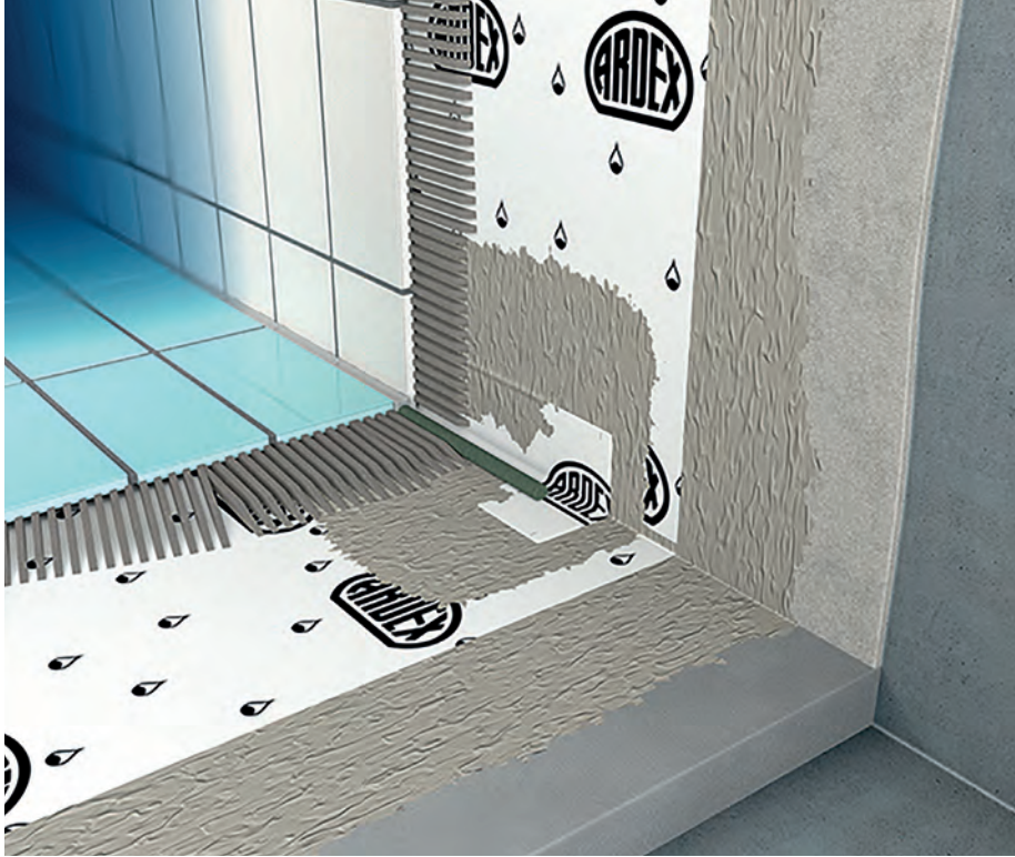
Duvar ve zemin birleşme kenarları uygulama kesiti
