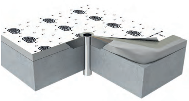
Su gideri uygulama kesiti 1
